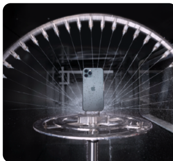
For at teste for IPX3/4-vandafvisning bruger Apple en svingarm med dyser til at simulere spray eller sprøjt med vand på iPhone.
